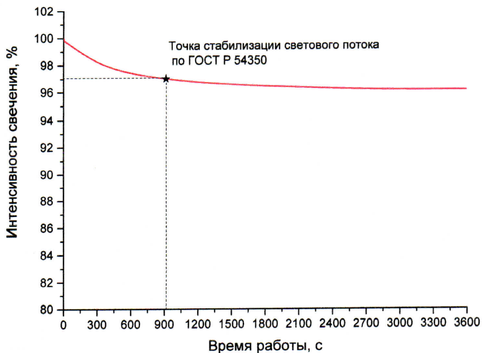
Рисунок 3 – График стабилизации светового потока образца светильник светодиодный Geniled Optimus 3Mx1L 60Вт 5000К III
