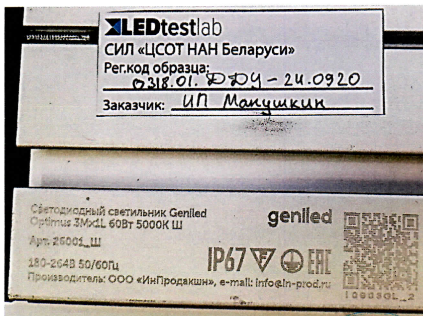
Рисунок 5 – Фотографии образца светильник светодиодный Geniled Optimus 3Mx1L 60Вт 5000К Ш
