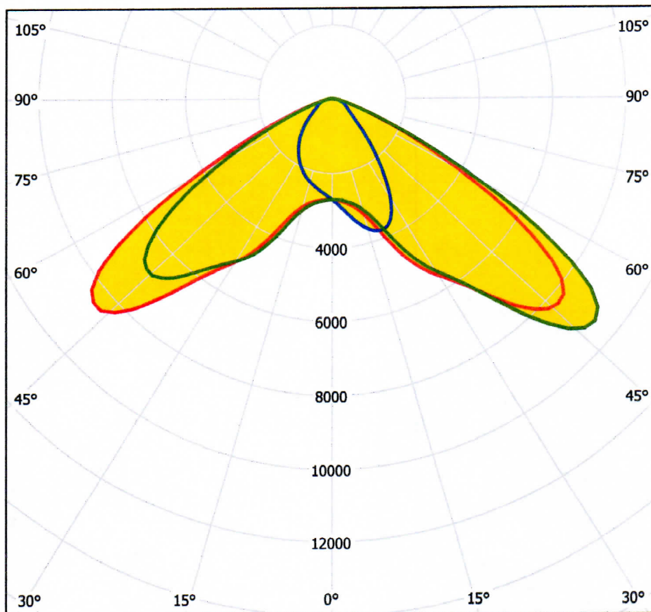
Рисунок 1 – КСС образца светильник светодиодный Geniled Optimus 3Mx1L 60Вт 5000К III в поперечной (C0-C180) (красная кривая), продольной (C90-C270) (синяя кривая) плоскостях и плоскости максимальной силы света (C174-C354) (зеленая кривая)
