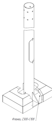
Рисунок 2а. Составные части на примере стойки основания Geniled Park C108-4000-z300
