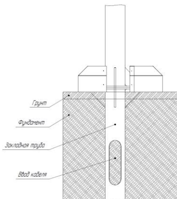
Рисунок 2б. Установка декоративной накладки на примере трубной закладной Z300-1000-C108
