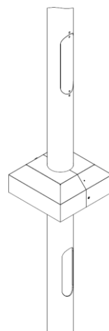
Рисунок 2г. Вид смонтированного изделия на примере декоративной накладки Geniled Park N200-C108
