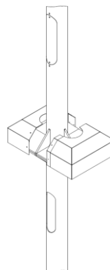
Рисунок 2б. Установка декоративной накладки на примере трубной закладной Z300-1000-C108
