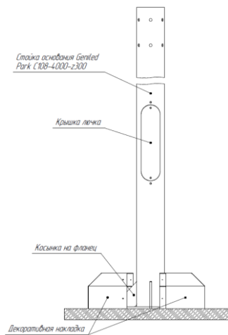
Рисунок 2а. Составные части на примере стойки основания Geniled Park C108-4000-z300
