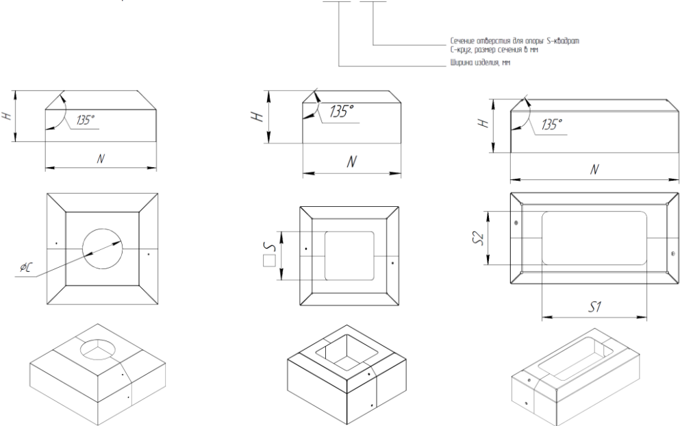
Рисунок 1. Габаритные размеры и виды декоративных накладок Geniled Park
