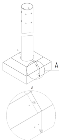
Рисунок 2в. Узел крепления половинок накладки на примере декоративной накладки Geniled Park N200-C108
