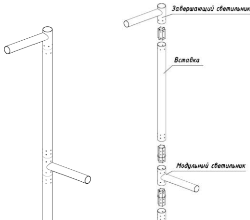
Рисунок 2. Положение вставки Geniled Park C108 в опоре на примере светильника Geniled Park Torus.
