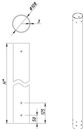
Рисунок 1. Габаритные размеры вставки Geniled Park C108.
