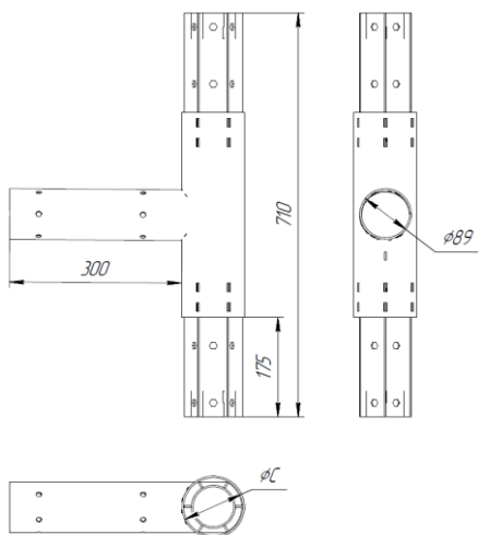
Рисунок 4. Габаритные размеры М-консоли для светильника Geniled Park Saturn CXX-XXX-CXXX.
