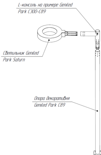
Рисунок 3. Положение L-консоли для светильника Geniled Park Saturn на стойке основания.
