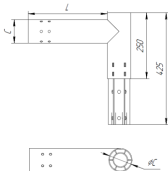
Рисунок 2. Габаритные размеры L-консоли для светильника Geniled Park Saturn CXX-XXX-CXXX.
