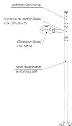
Рисунок 5. Положение М-консоли для светильника Geniled Park Saturn на стойке основания.
