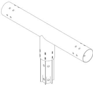
Twin-консоль для светильника Geniled Park Saturn
