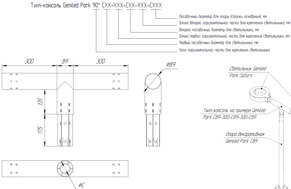
Рисунок 6. Габаритные размеры Twin-консоли для светильника Geniled Park Saturn CXX-XXX-CXX-XXX-CXXX.
