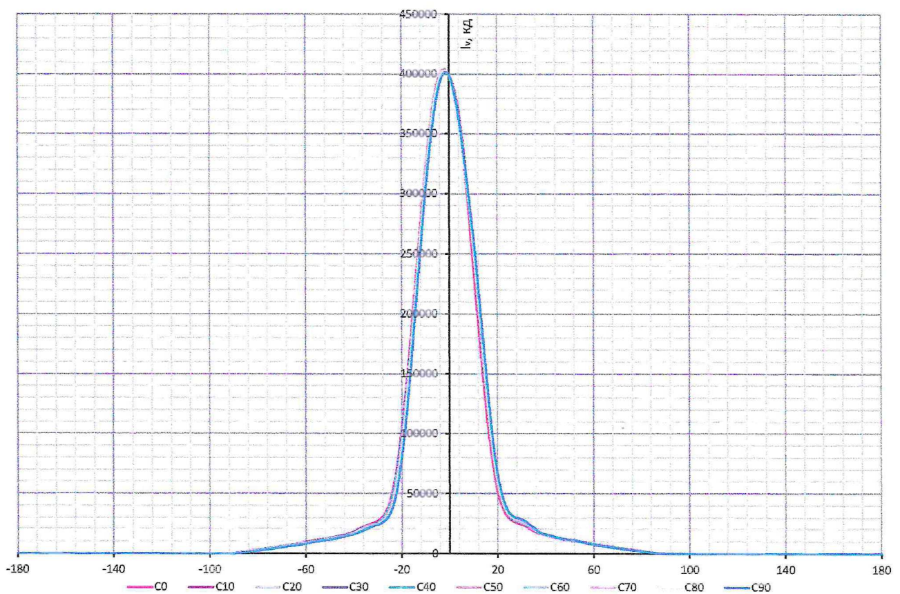
Рисунок 2. Декартовы координаты
