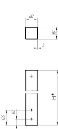
Рисунок 1. Габаритные размеры вставки Geniled Park S80.
