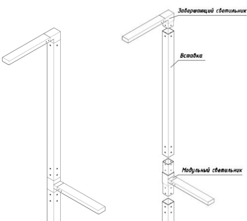
Рисунок 2. Положение вставки Geniled Park S80 в опоре на примере светильника Geniled Park Aist.
