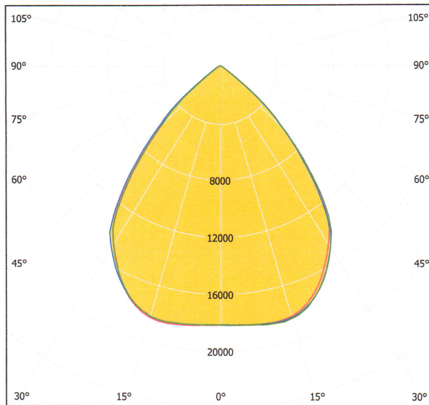
Рисунок 1 – КСС образца светильник светодиодный Geniled Kolokol 200Вт 5000K 80Ra , Закаленное стекло 120° с диффузором алюминиевым 90° в поперечной (C0-C180) (красная кривая), продольной (C90-C270) (синяя кривая) плоскостях и плоскости максимальной силы света (C128-C308) (зеленая кривая)
