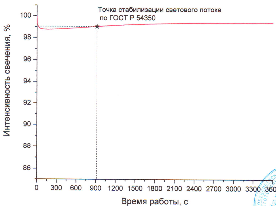
Рисунок 2 – График стабилизации светового потока образца светильник светодиодный Geniled Kolokol 200Вт 5000K 80Ra , Закаленное стекло 120° с диффузором алюминиевым 90°
